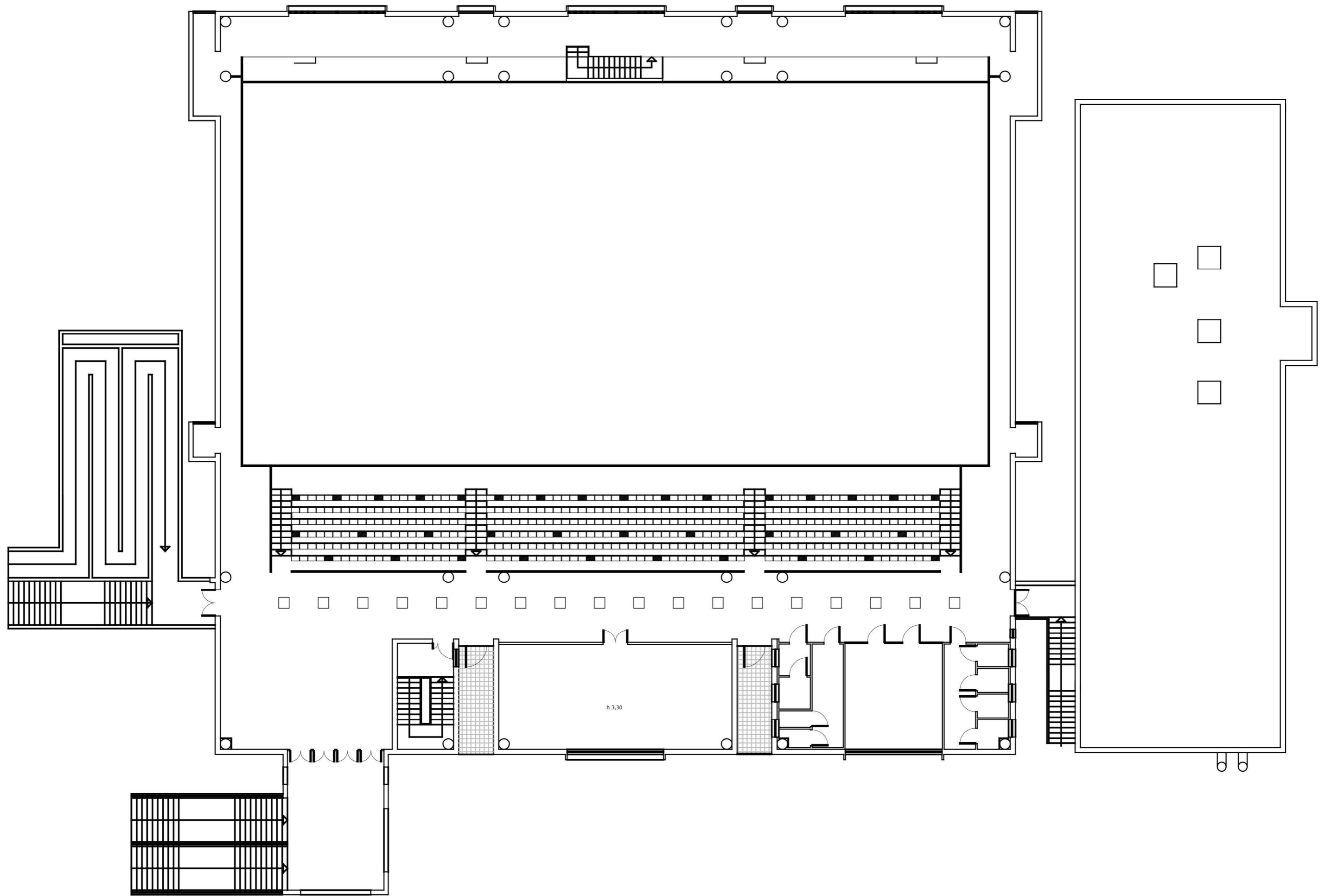
PALESTRA DI FONTANE - PIANO TRIBUNE
