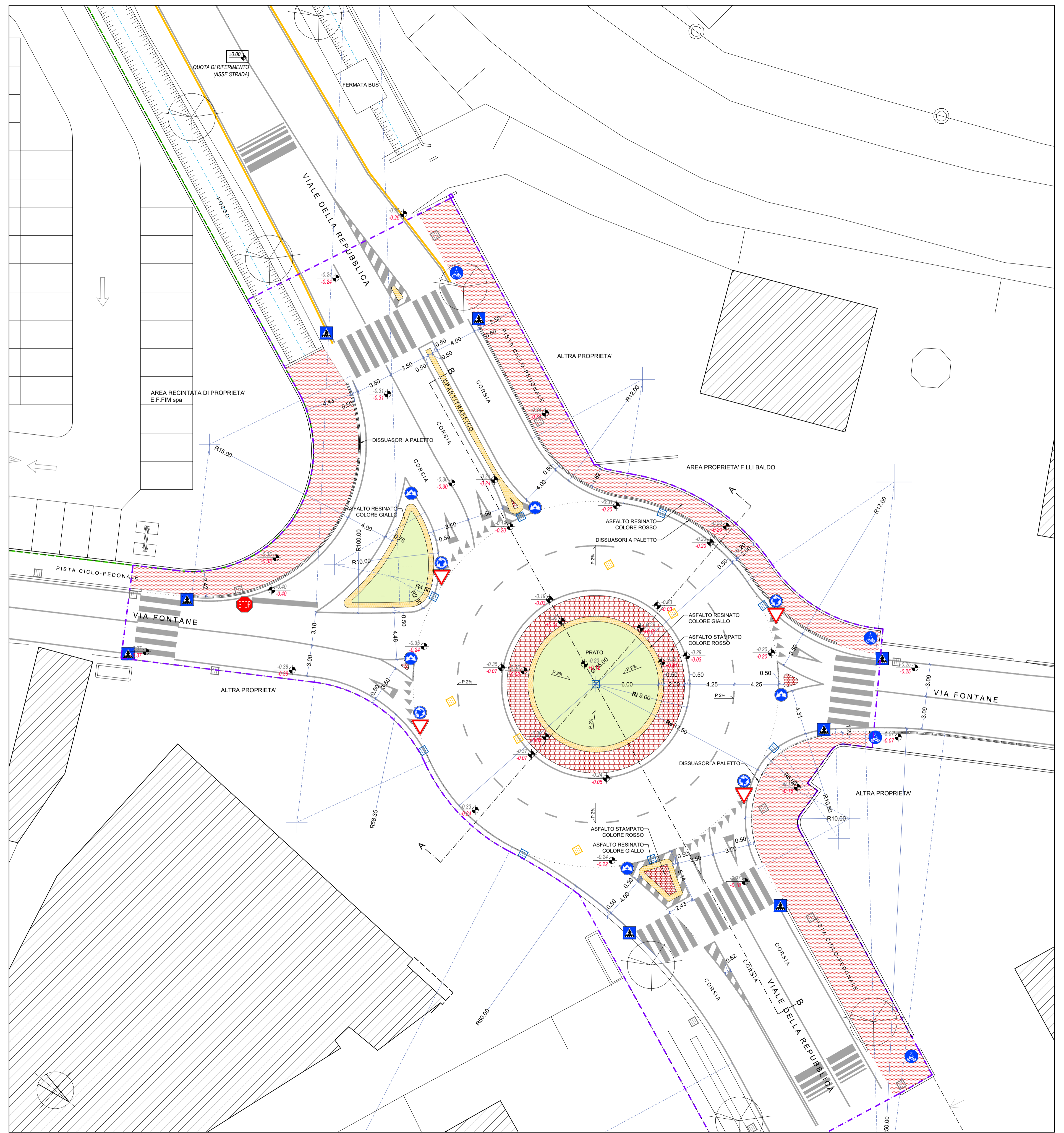
PLANIMETRIA - scala 1:200
