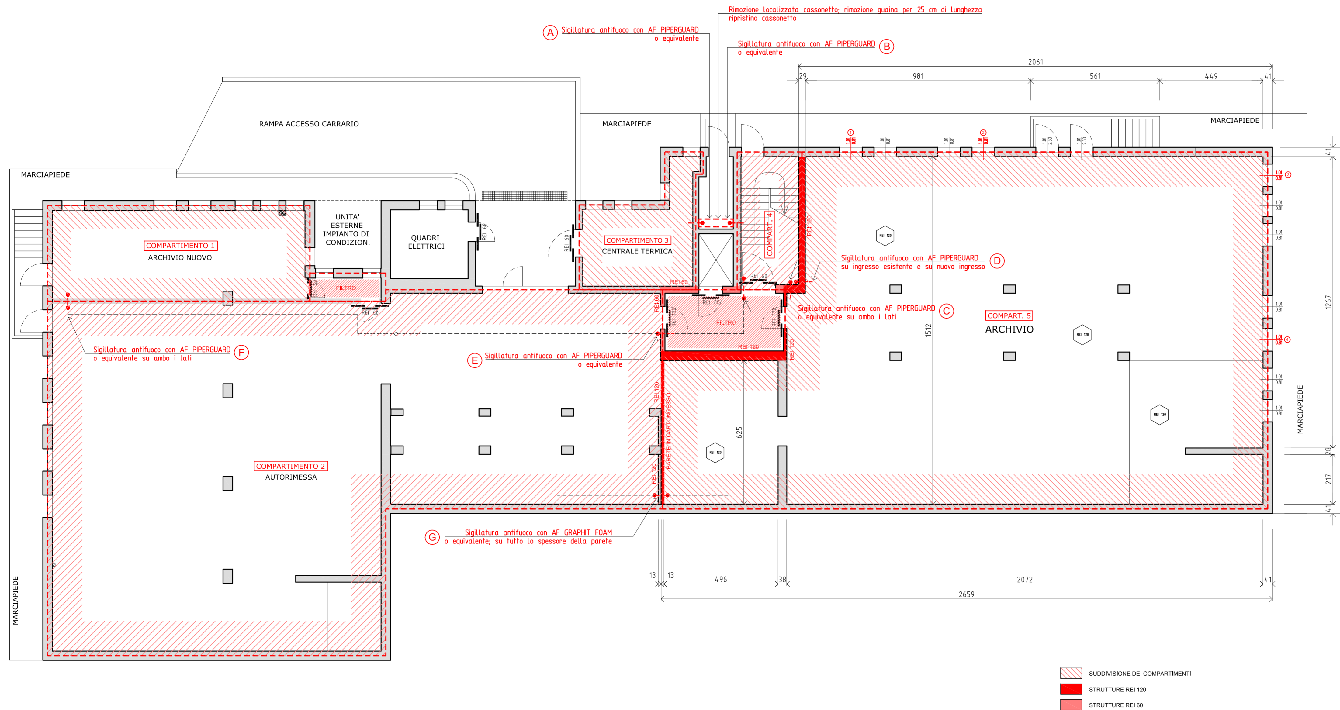
PIANTA PIANO SEMINTERRATO E LOCALI ACCESSORI 1/100
