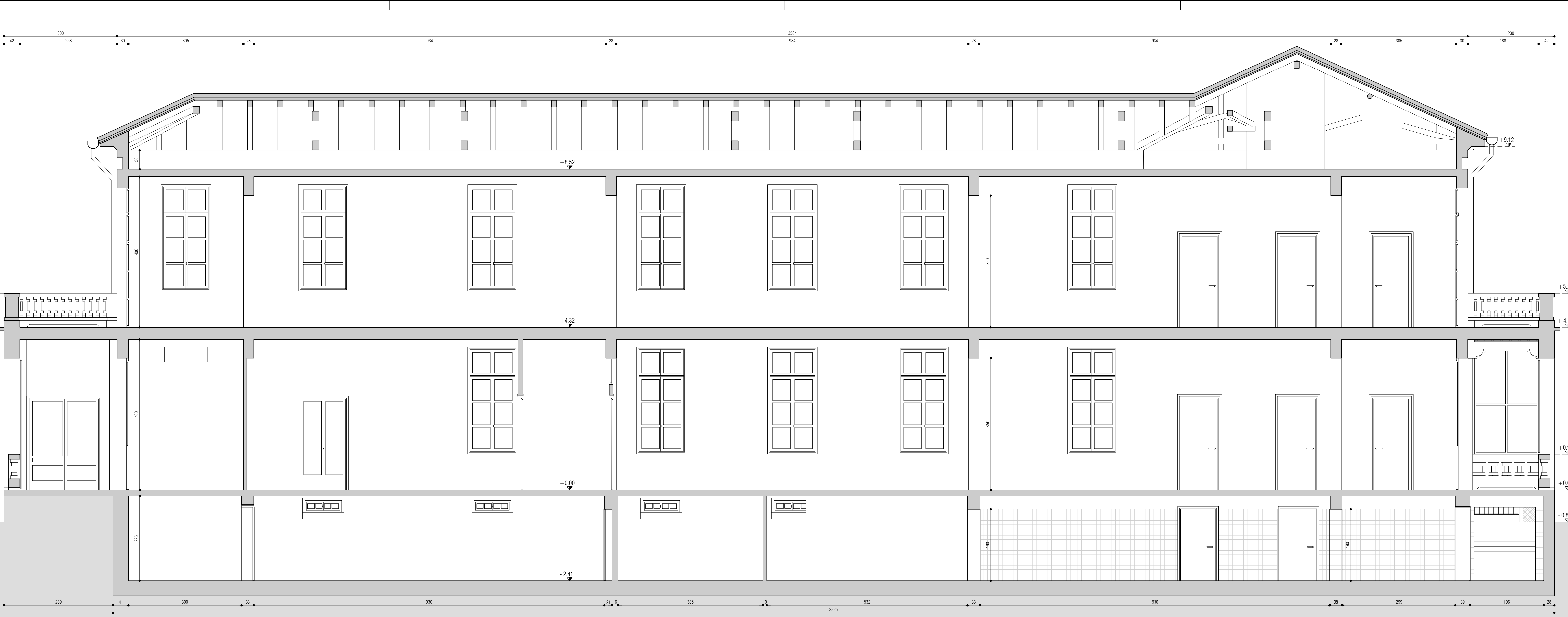
SEZIONE E-E
