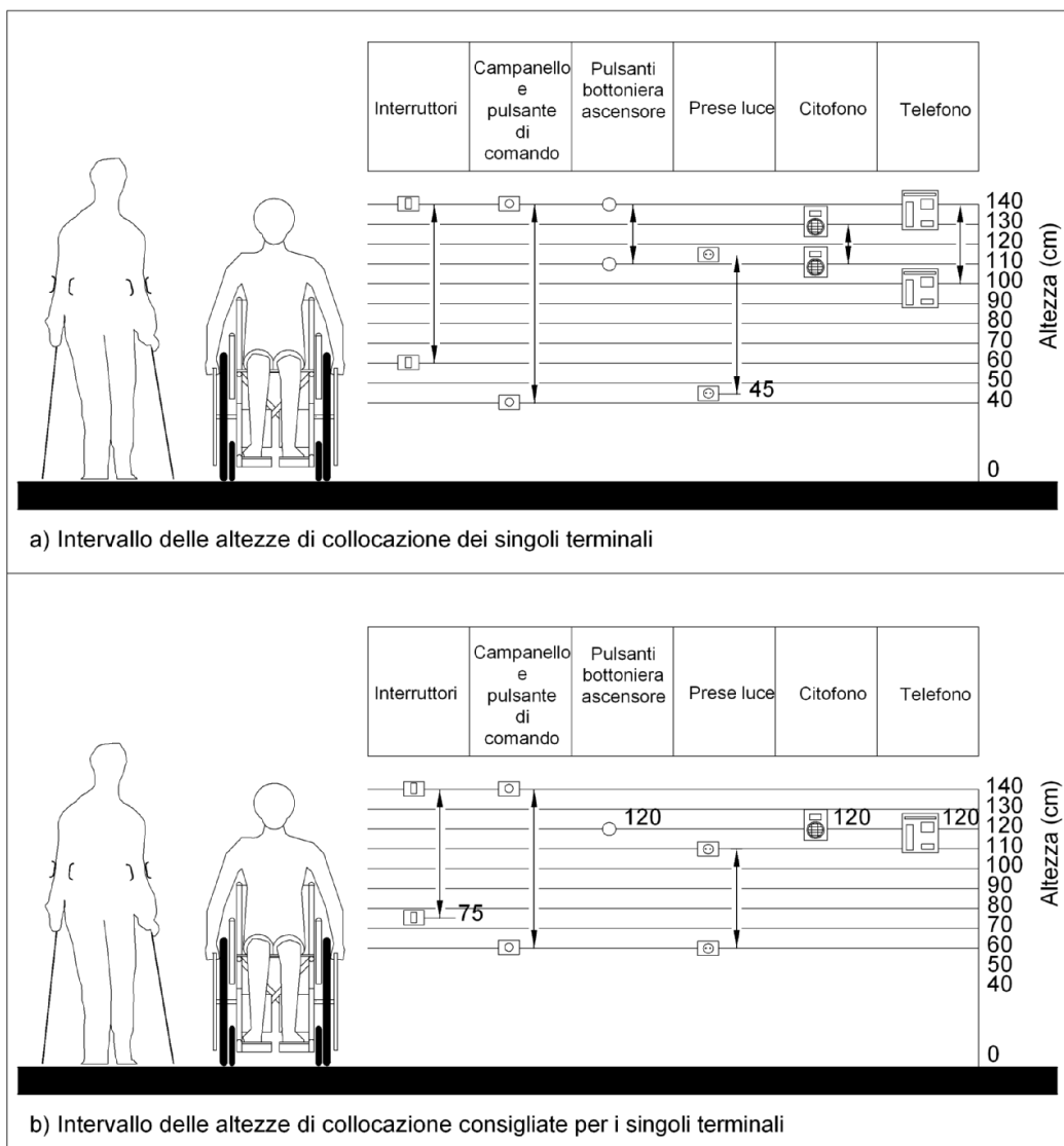
Figura 84.2 Altezze consigliate per i terminali degli impianti elettrici e telefonici
