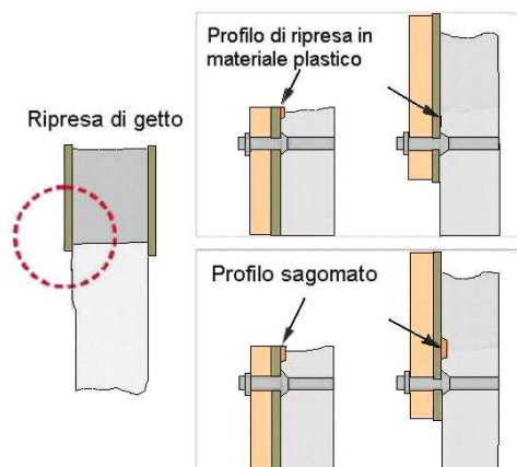
Figura 58.8 - Giunti delle casseforme in evidenza
