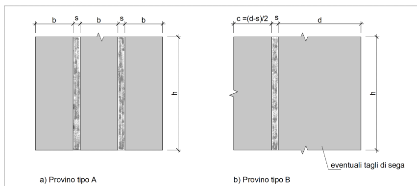
Figura 19.5 Dimensioni dei provini di muratura per prova, per la determinazione sperimentale della resistenza a taglio (riferimento UNI EN 1052-3)
