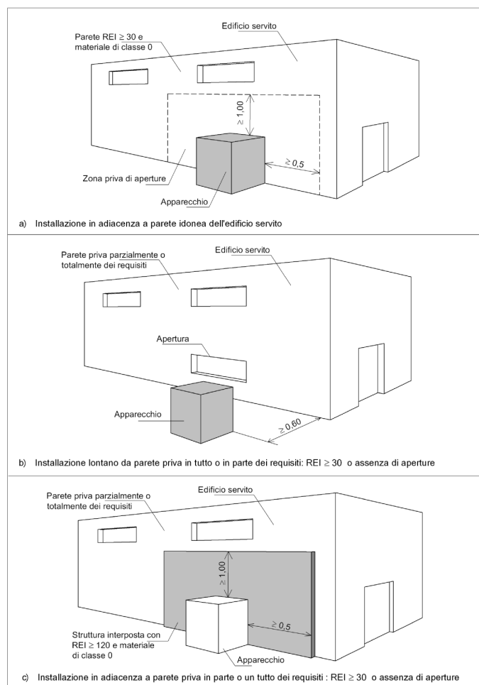
Figura 81.2 - Installazione degli apparecchi all'aperto
