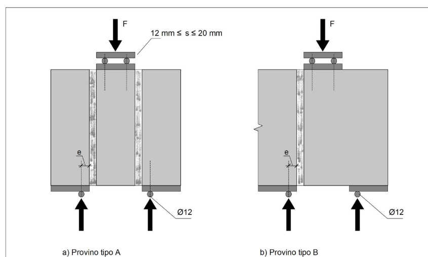
Figura 19.6 Carico di prova per la determinazione sperimentale della resistenza a taglio (riferimento UNI EN 1052-3)
