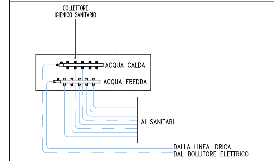
SCHEMA COLLETTORE IDRICO
