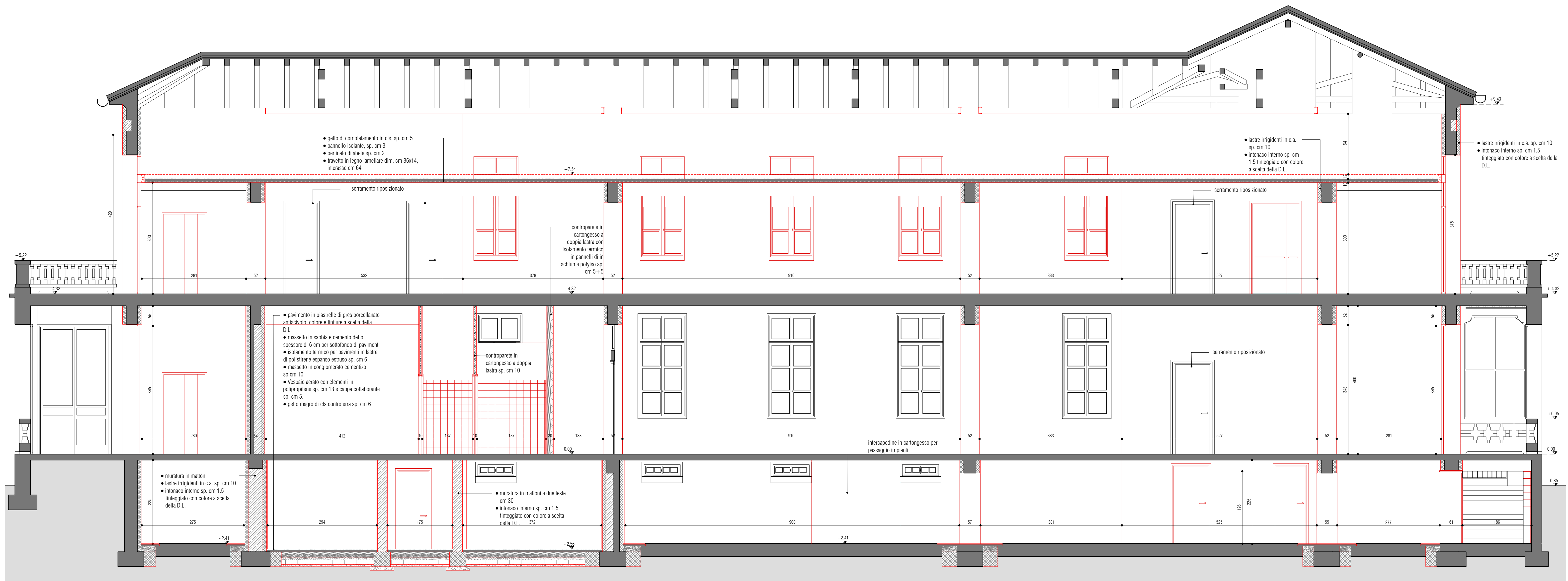
SEZIONE E-E
