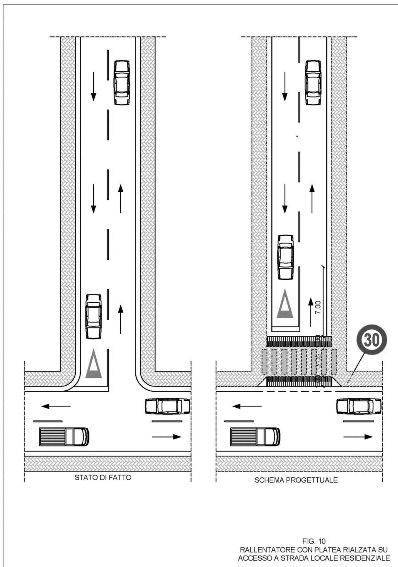
Figura 10 Rallentatore con platea rialzata su accesso a strada locale residenziale
