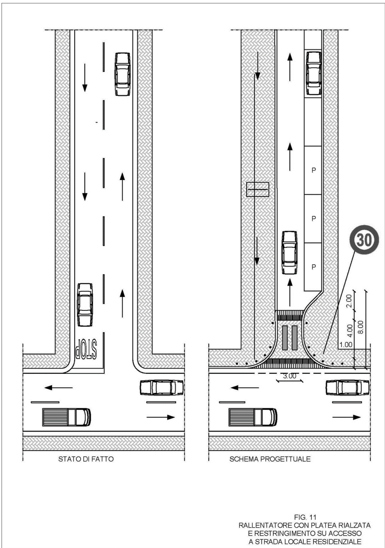
Figura 11 Rallentatore con platea rialzata e restringimento su accesso strada locale residenziale
