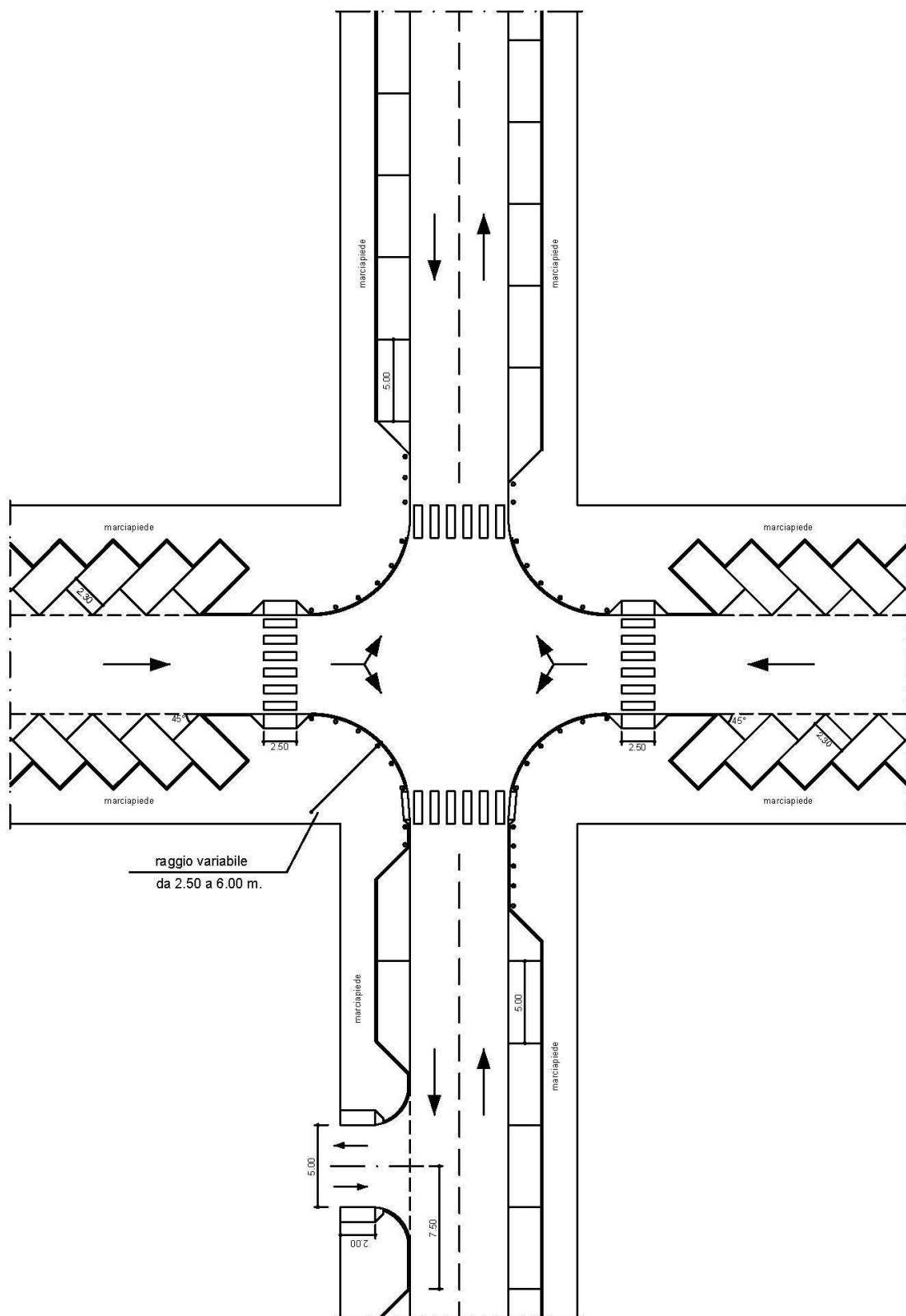
FIG. 6 SOLUZIONE TIPO DELLA SOSTA SU SEDE STRADALE IN PROSSIMITA' DEGLI INCROCI
