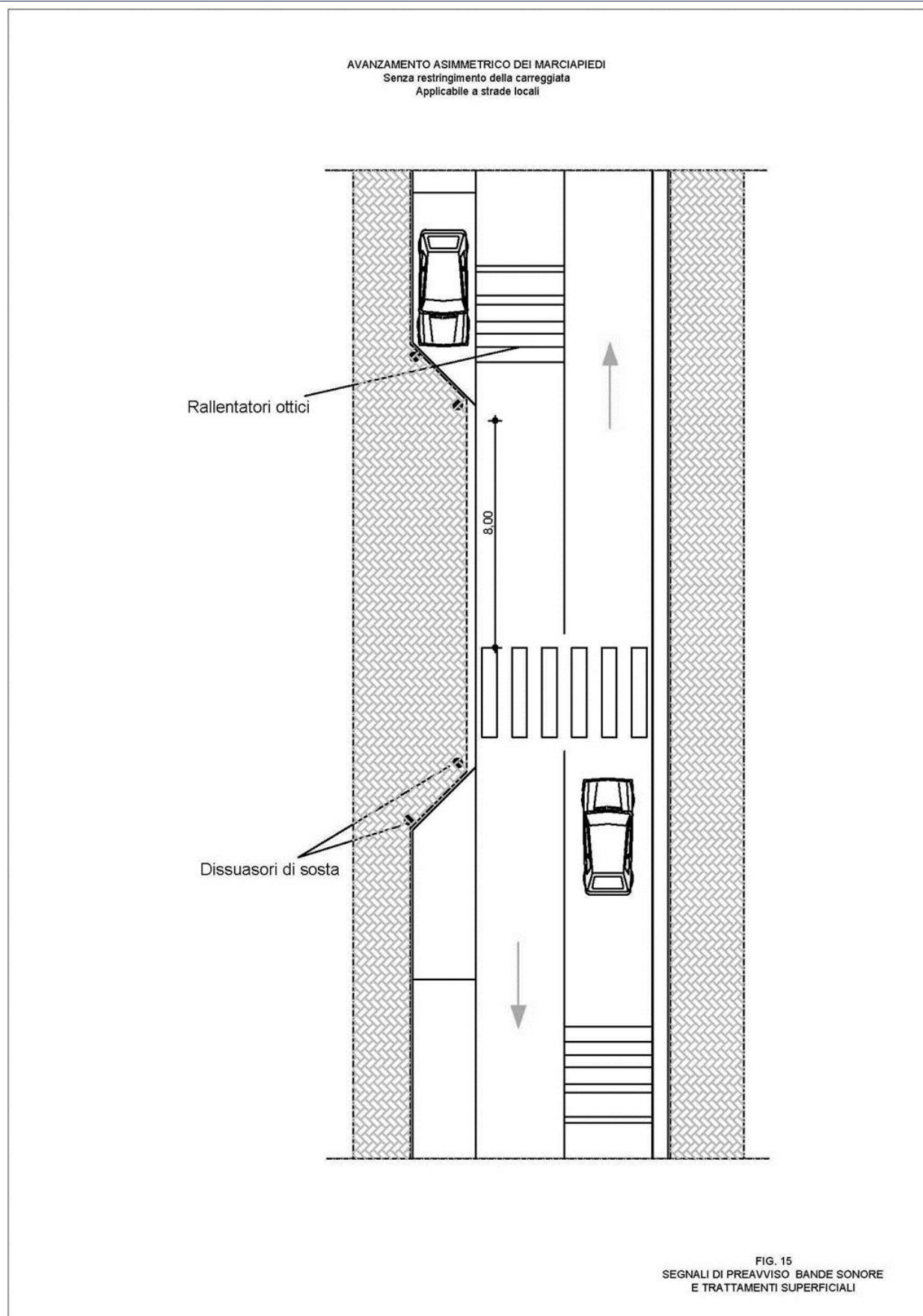
Figura 15 Segnali di preavviso bande sonore e trattamenti superficiali
